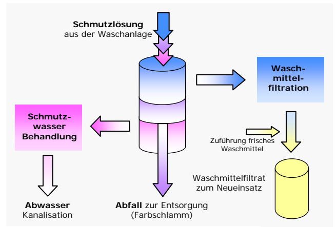
Abbildung: Waschmittel-Filtration
